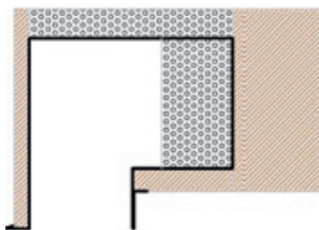
Rollokasten
